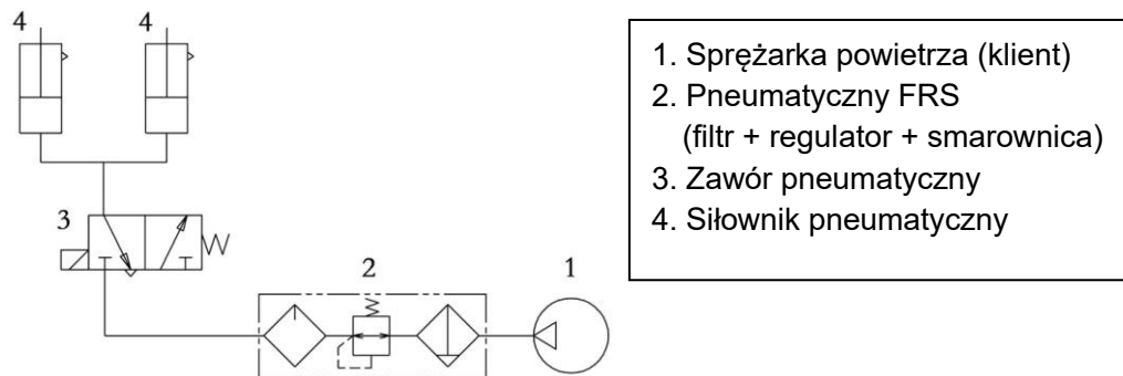
Rys. 9 Schemat układu pneumatycznego
