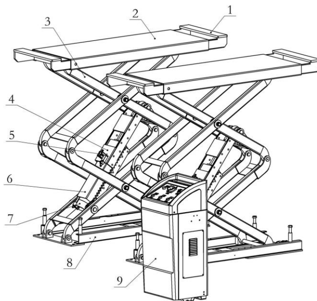
Rys. 1 Konstrukcja podnośnika
