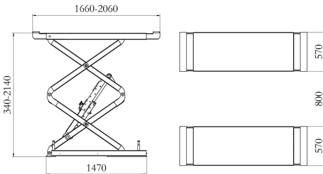
Rys. 2 Rysunek wymiarowy
